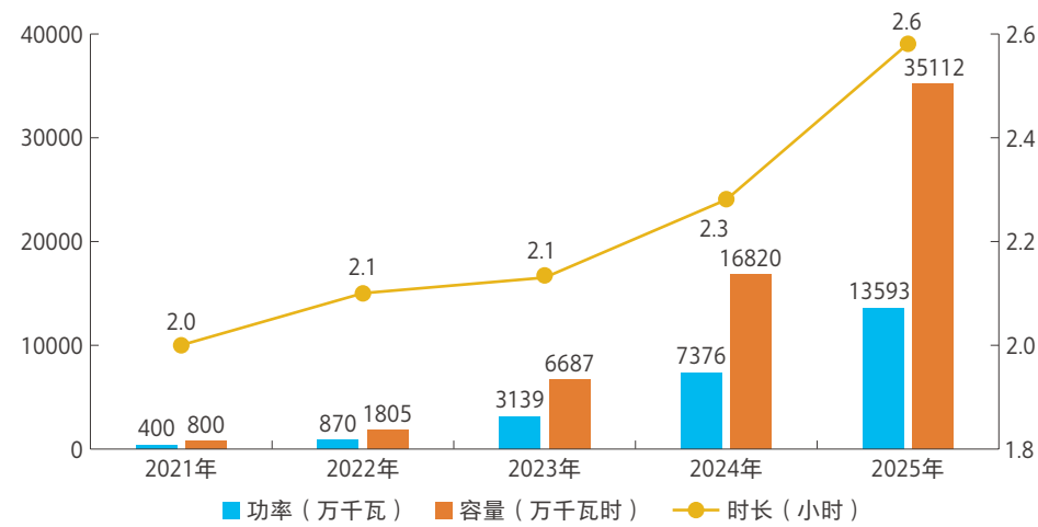
图 19 “十四五”以来我国新型储能装机规模情况
