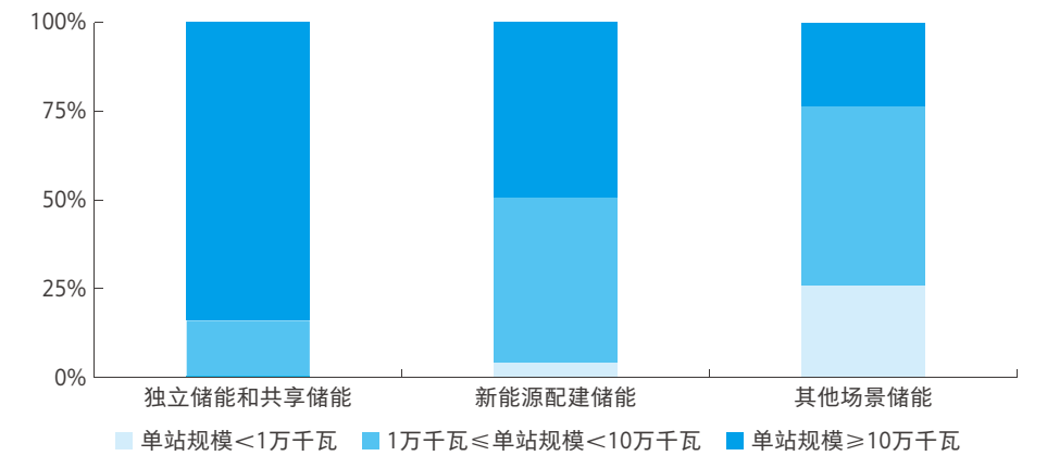
图 10 各应用场景下新型储能规模分布情况
